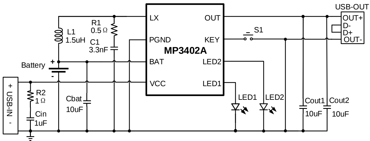
MP3402A 典型应用电路
